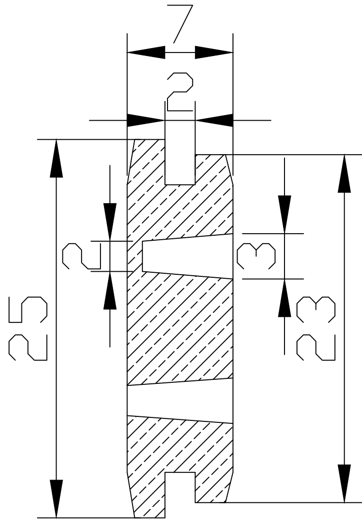
Sezione A-A
